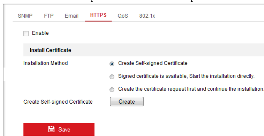
Obrázek 7–10 Okno konfigurace protokolu HTTPS
