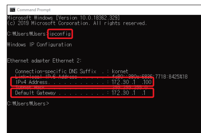
<okno cmd>
