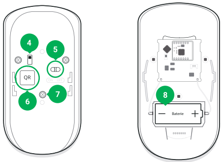
4 - Sabotážní kontakt 5 - Přepínač pro vypnutí / zapnutí 6 - QR kód 7 - Vruty pro zajištění krytu detektoru
