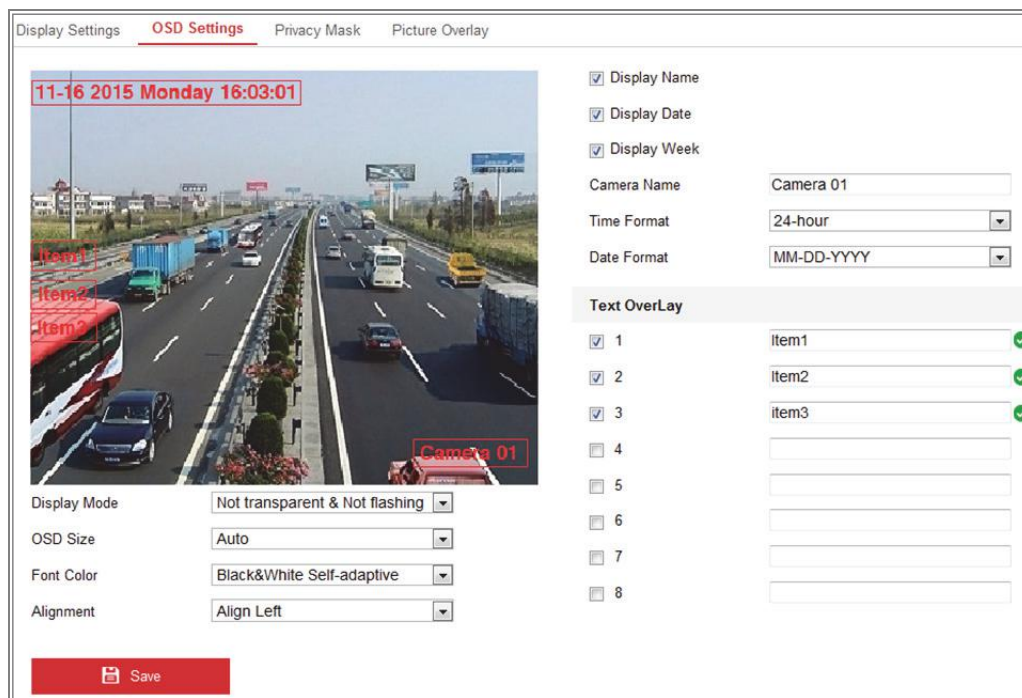
Obrázek 9-6 Nastavení OSD
