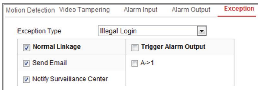
Obrázek 10-9 Nastavení výjimky
