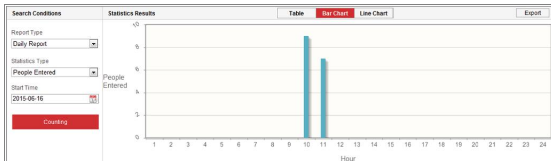
Obrázek 14-2 Počítání lidí
