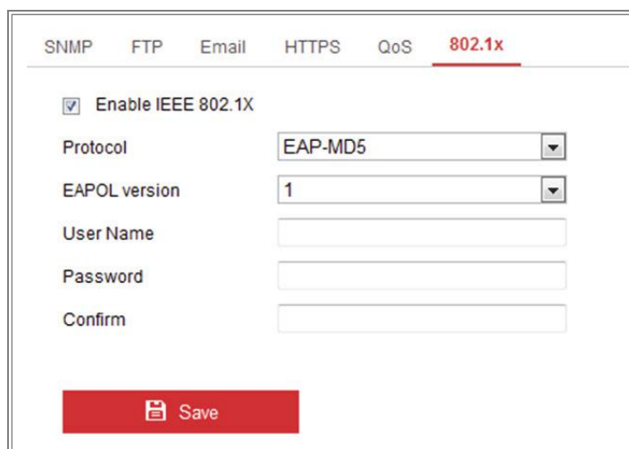
Obrázek 7-14 Nastavení 802.1X
