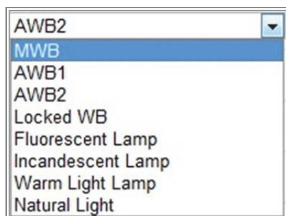
Obrázek 9-4 Vyvážení bílé
