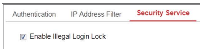
Obrázek 6-19 Služba zabezpečení
