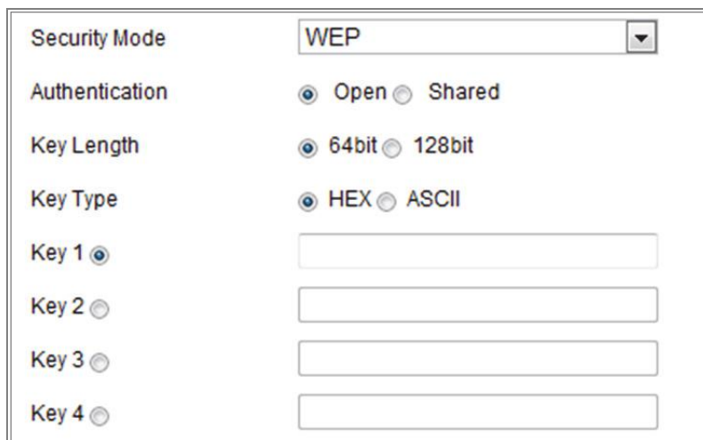
Obrázek 4-6 Režim WEP
