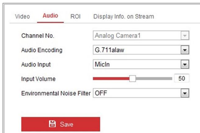
Obrázek 8-3 Nastavení zvuku
