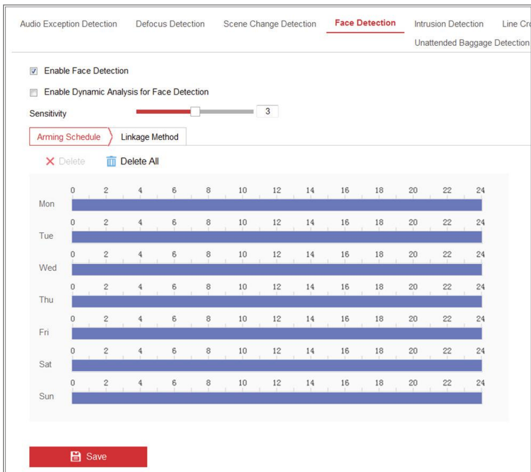
Obrázek 10-18 Detekce obličeje
