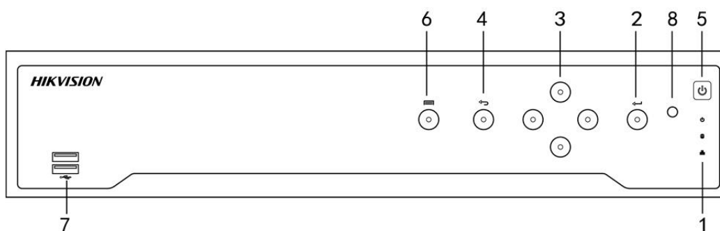
Obrázek 1–4 Řada DS-8600NI-K8
